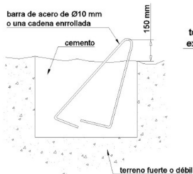
Anclaje de fácil fabricación
